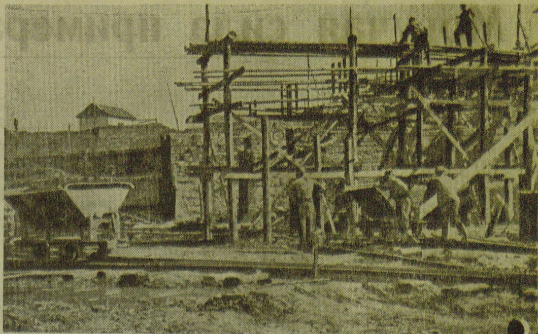
На головном сооружении. Раздельный бык плотина одевается в гранит. На снимке: подготовка для производства гранитной облицовки. Фото З. Луденского.
